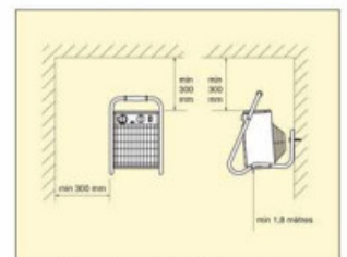
Fig. 1: Distances de sécurité pour une installation fixe.
