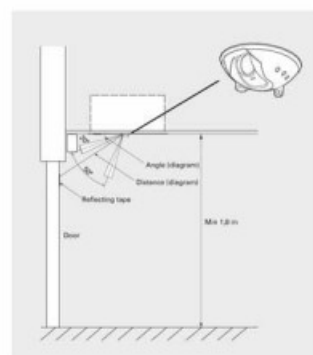
Fig. 1: Réglages de hauteur du capteur IR et distance minimale du sol.
